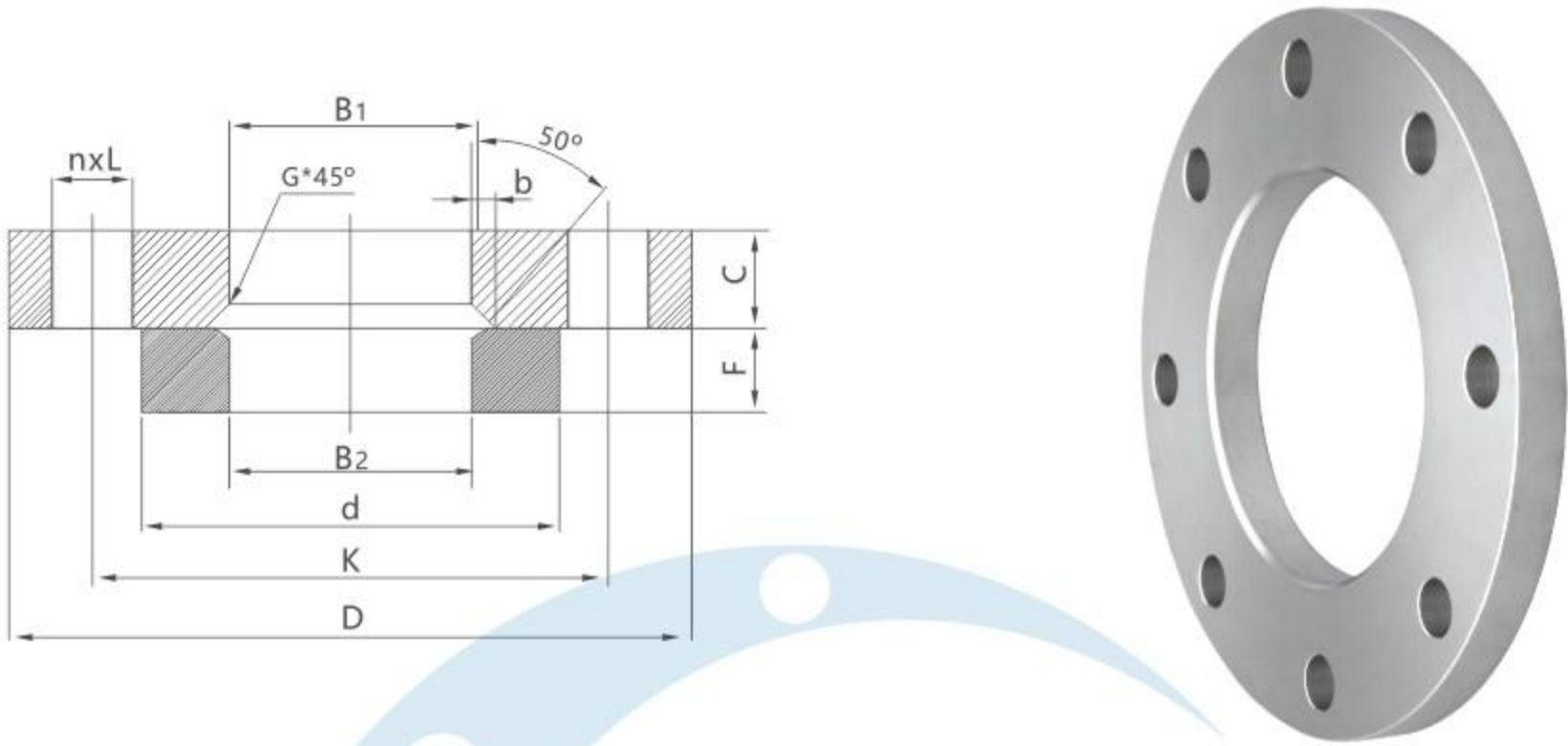
PN6 平焊环松套钢制管法兰
