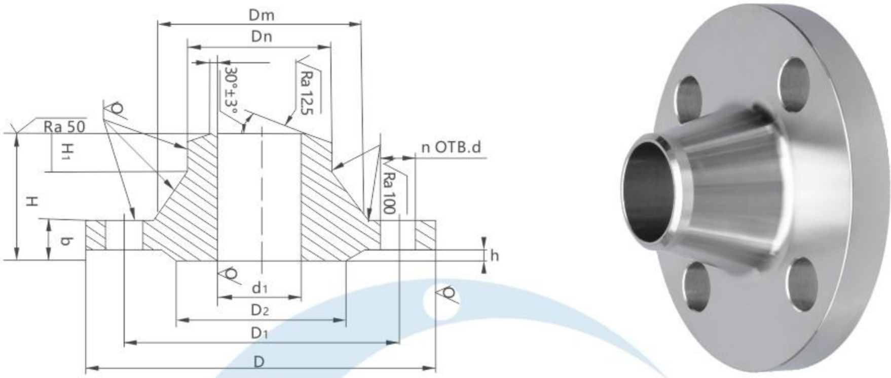
PN0.6 GOST 33259-2015 Type 01 Char.B
