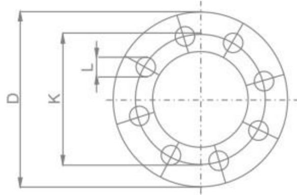
Dimensions of PN 16 Flanges EN 1092-1
