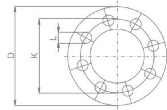
Dimensions of PN 16 Flanges EN 1092-1
