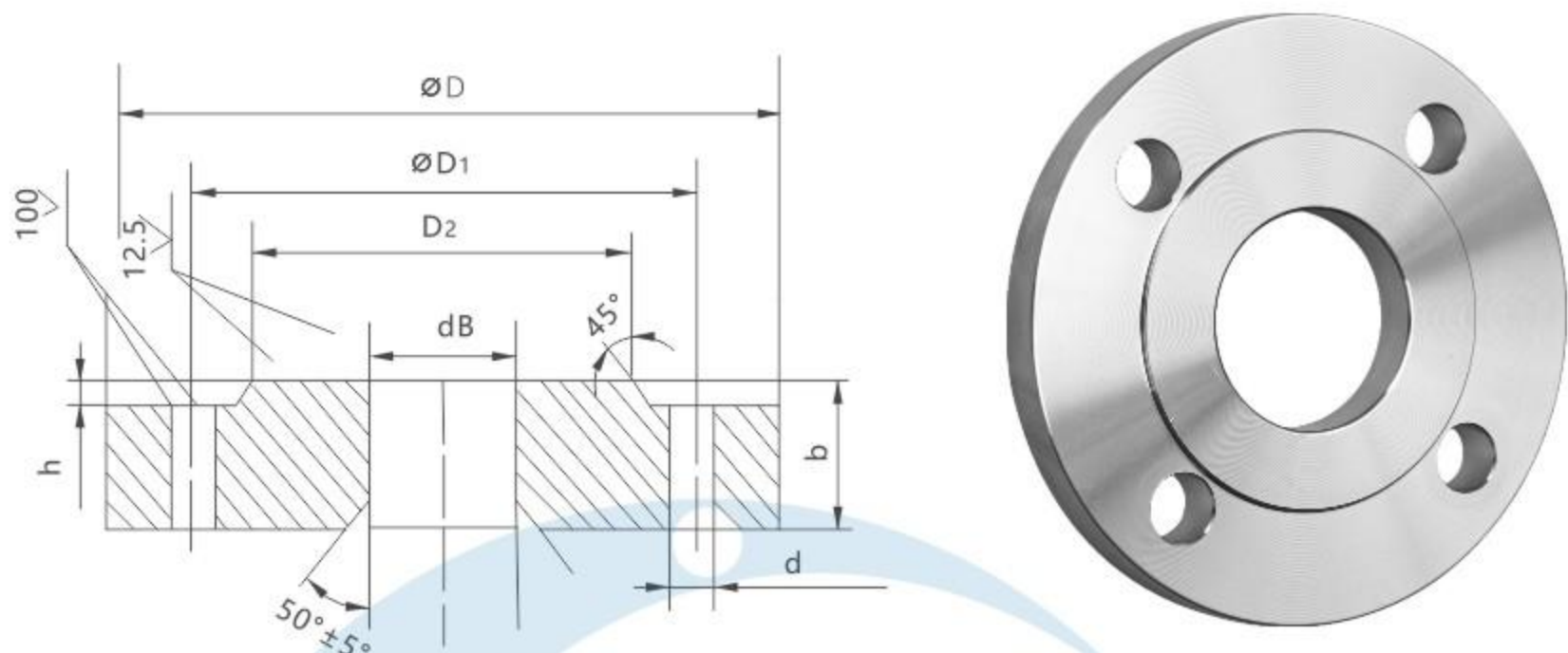
PN6 GOST 33259-2015 Type 01 Char.B
